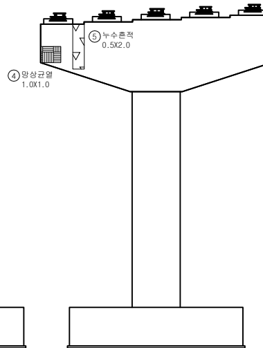
배면
